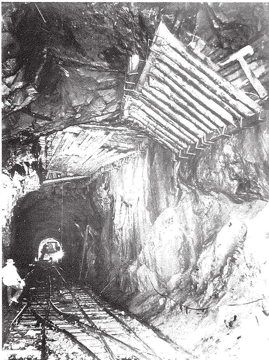
Arbeidet i den lange Kvinesheitunnelen var farefullt. Fjellet var dårleg mange stader, og måtte sikrast for ikkje å rase ut. Dei sikra partiene vart seinare mura til.
